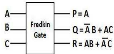
Figure 8. Fredkin Gate. Source: (H. Thapliyal, et al).
