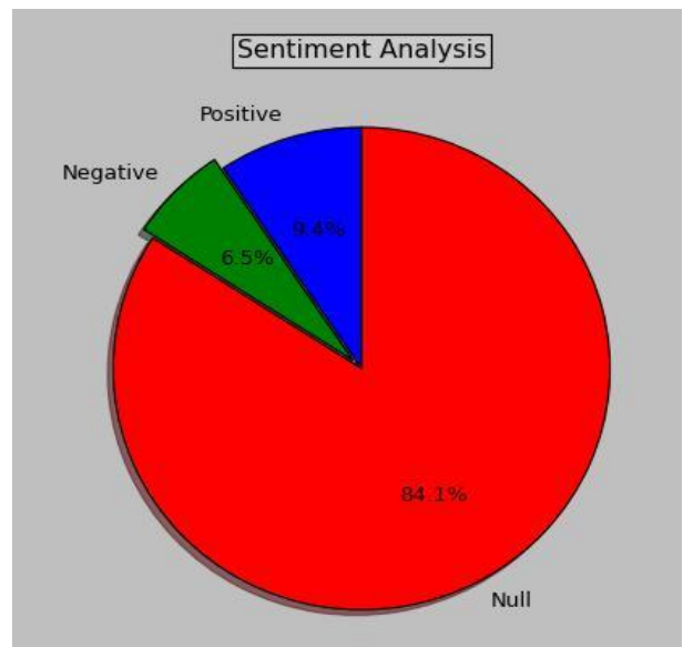
Fig. 1. Pie Chart
